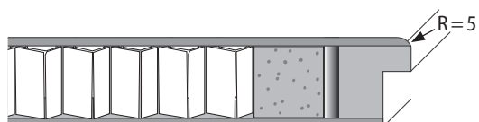
QUERSCHNITT TÜRBLATT
