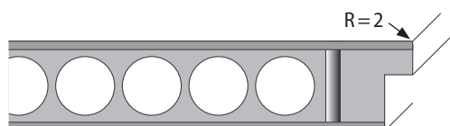
QUERSCHNITT TÜRBLATT
