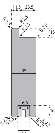
Riegel oben
