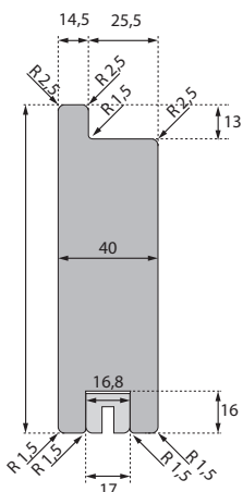
Riegel seitlich
