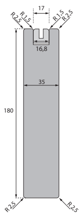
Sockel
