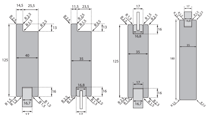
Riegel seitlich
